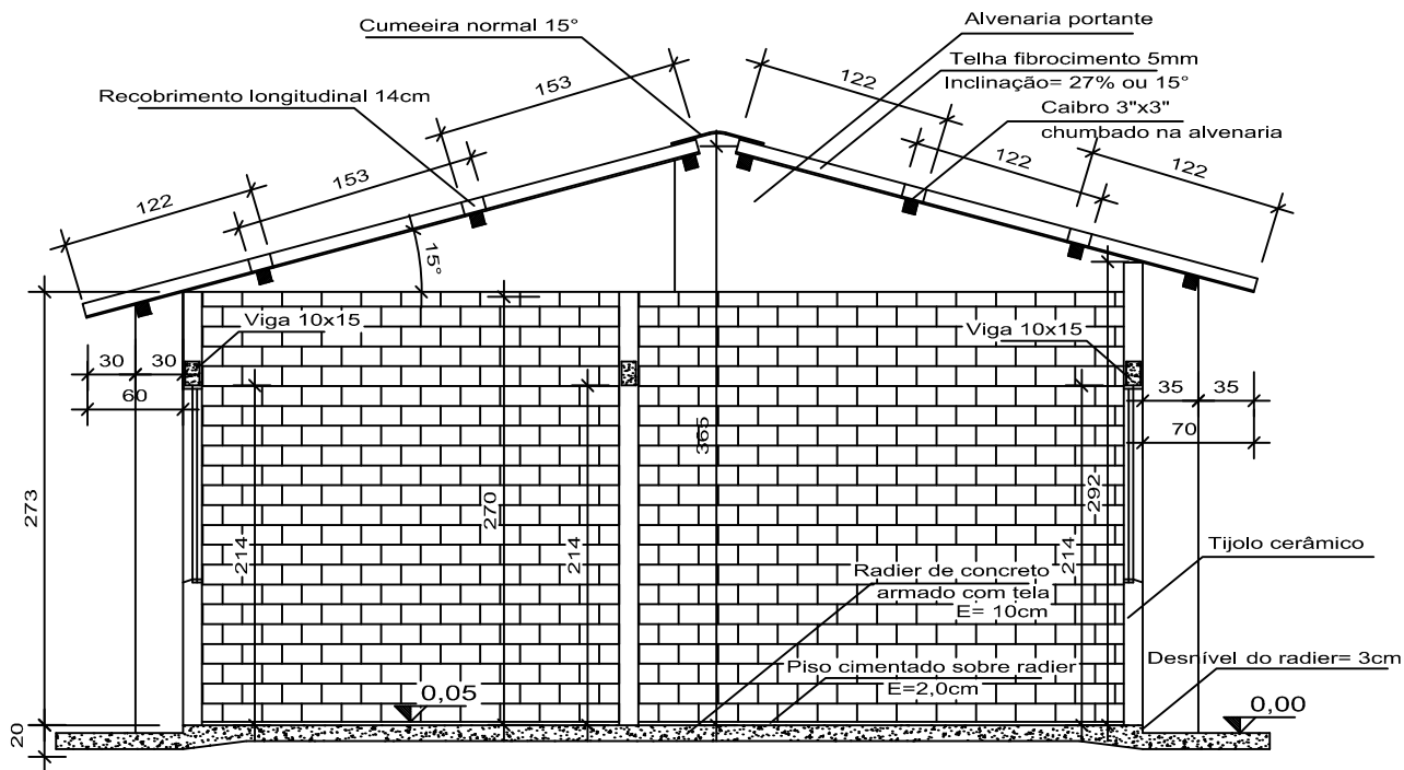
CORTE AA
