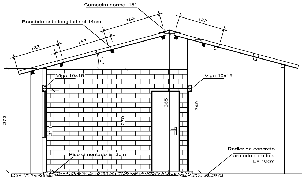
CORTE AA
