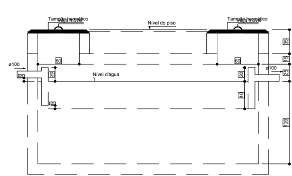
Tanque séptico Corte 1 - ESC. 1:25
