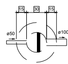
Caixa de gordura Planta baixa - ESC. 1:25
