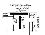
Caixa de gordura Corte 1 - ESC. 1:25
