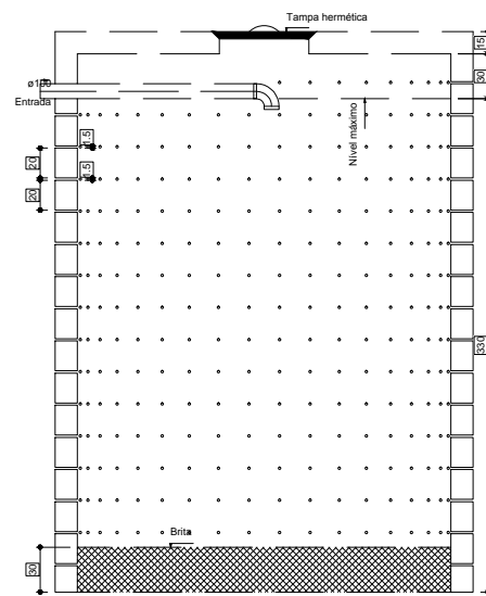
Sumidouro Corte 1 - ESC. 1:25
