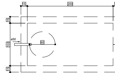
Tanque séptico 2 Planta baixa - ESC. 1:25
