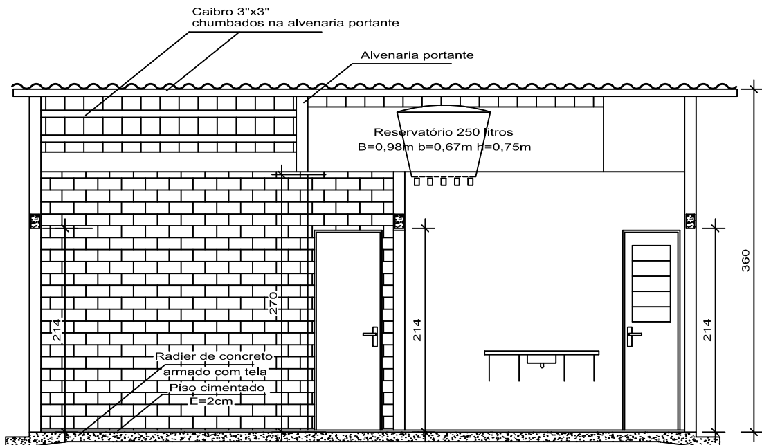
CORTE CC
